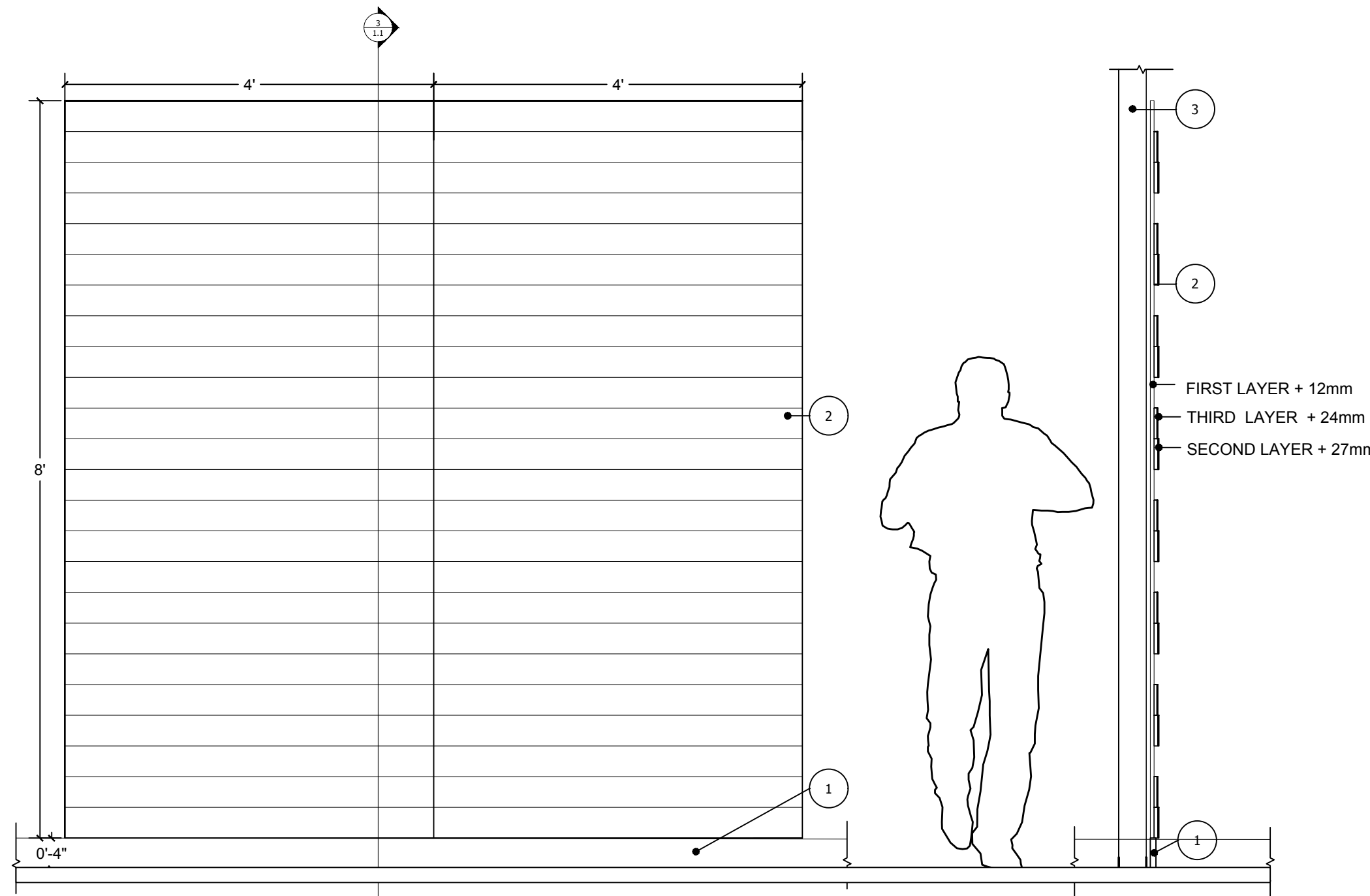
4 SLAT DEPTH ELEVATION Scale: 3/4" = 1'-0"
